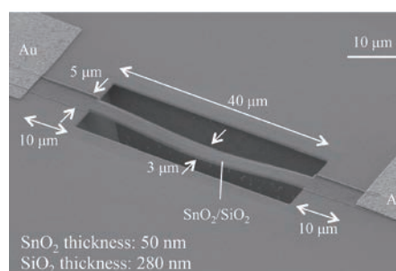
ナノメカニカル振動子
