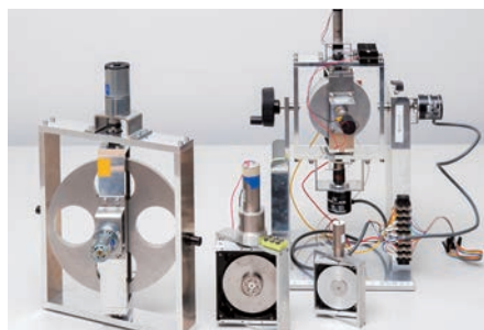
ジャイロ効果を用いる振動発電機
