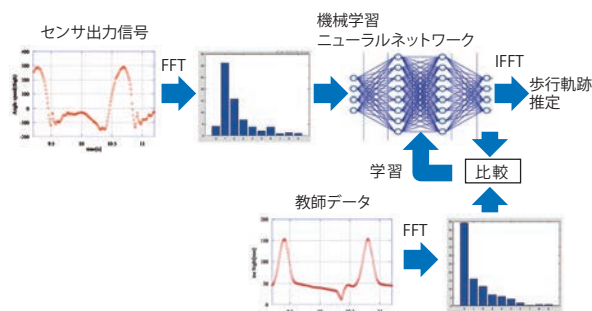
図4 システム制御方法と機械学習を用いたつま先歩行軌跡推定
