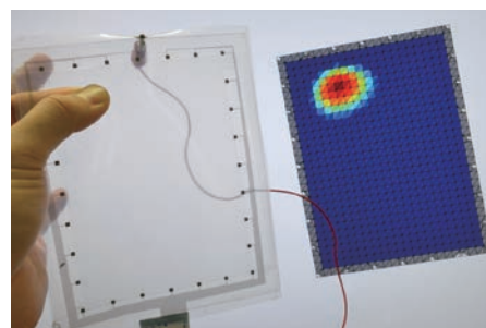
トモグラフィを用いた触覚センサ
