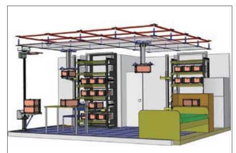
家庭内物流支援ロボットシステム
