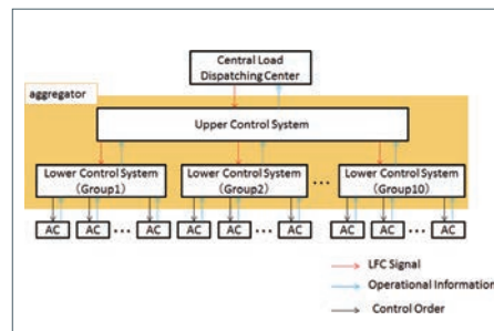
空調機を用いたスマートグリッドの階層制御構造
