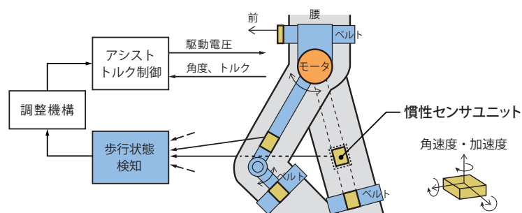
図2 超音波モータを用いた歩行アシストの制御方法
