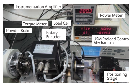
図3 予圧制御型超音波モータの実験装置
